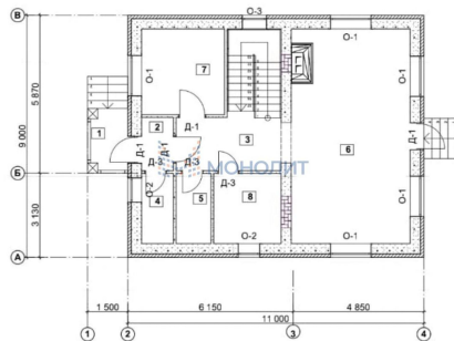
Экспликация помещений 1 этажа
