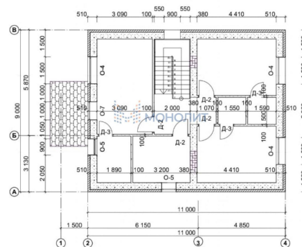
План 2 этажа
