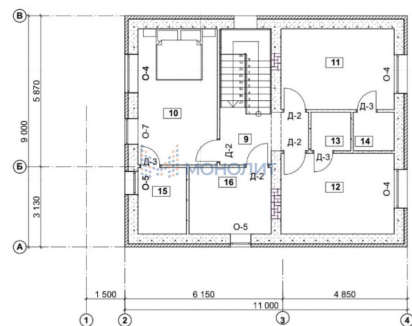
Экспликация помещений 2 этажа
