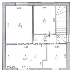
2 этаж
