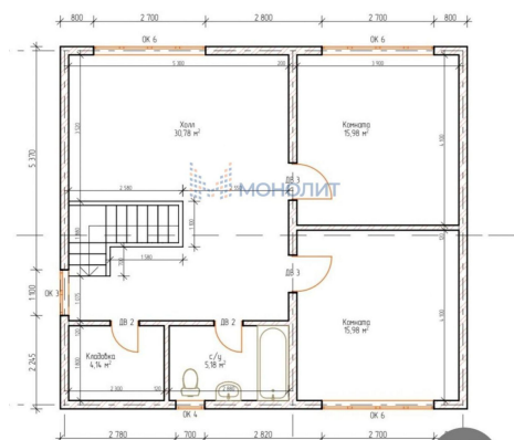
План на отметке +2.900
